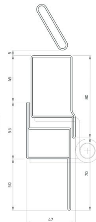
Nodo laterale Side node
