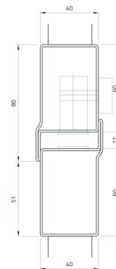
Nodo centrale Central node
