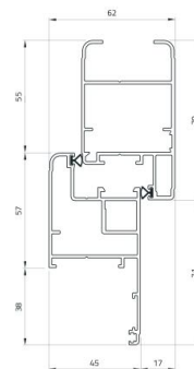
Nodo laterale Side node
