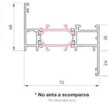
Telaio a ZETA 24 mm ZETA frame 24mm
