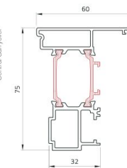
Riparto Centrale Central Crosspiece
