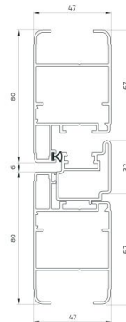
Nodo centrale Central node
