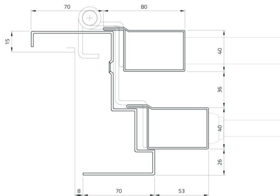
Nodo laterale Side node
