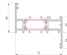
Telaio a ZETA 24 mm ZETA frame 24mm
