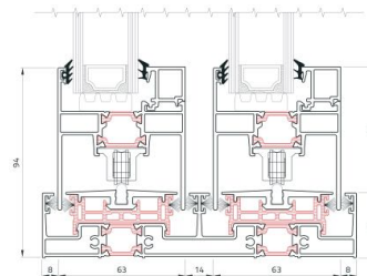
Sistema doppio binario Double track system
