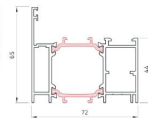
Telaio piano maggiorato Flat majorated frame
