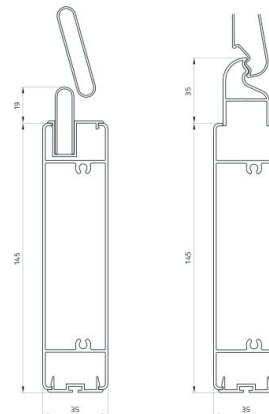
Nodo inferiore Bottom node
