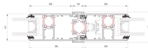
Sistema doppio binario Double track system
