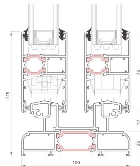
Sistema doppio binario Double track system
