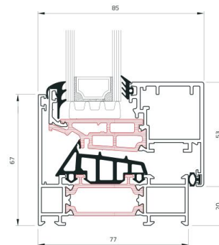
Sistema anta a scomparsa Retractable door system
