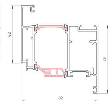
Anta Portoncino Ap. Interna Inward Opening Door Leaf
